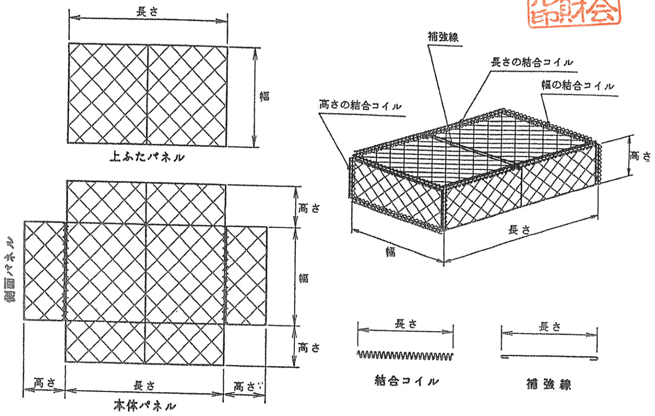
図3 パネル式角形じゃかごの形状及び各部の名称
