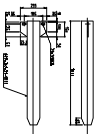
支柱用バネアンカー
