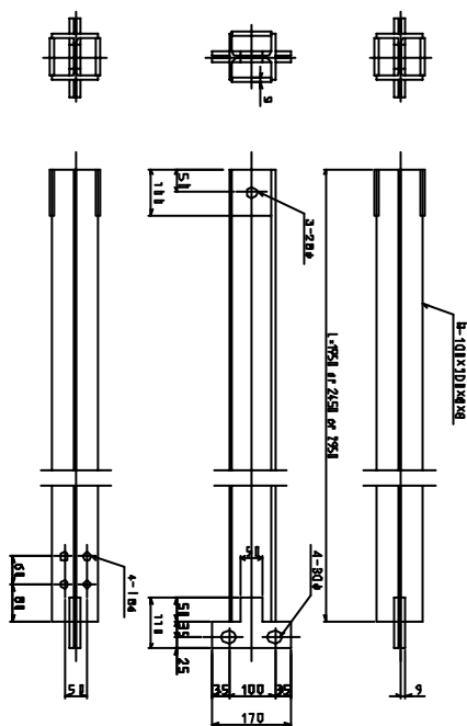
スクリュー
